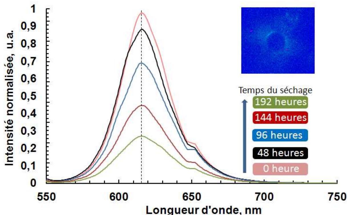
Figure 16 : Evolution des spectres d'émission enregistrés à la sortie de 20 cm de fibre en fonction du temps de traitement. En insert : champ proche mesuré à la sortie de la fibre.
