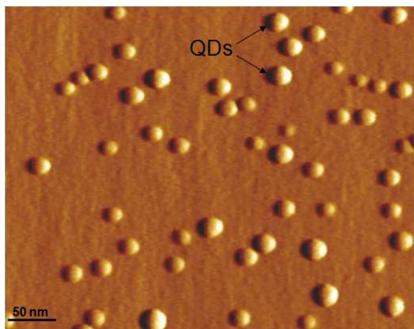
Figure 15 : QDs fabriqués par la technique épitaxie par jets moléculaires.
