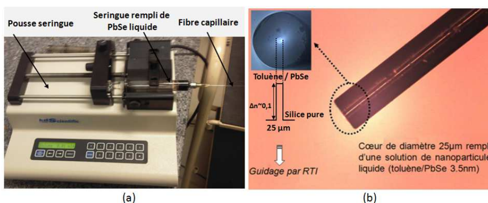
Figure 7 : (a) Remplissage d'une fibre capillaire de diamètre de cœur 25 \mu\text{m} à gaine silice par la solution liquide de nanoparticules (3,5 nm-PbSe dissoutes dans du toluène) à l'aide d'un pousse seringue ; (b) Coupe longitudinale de la fibre remplie. En insert : image optique de la fibre couplée en transmission à une source de lumière blanche et son profil équivalent à saut d'indice (ouverture numérique estimé \sim 0,1 ).
